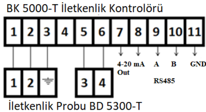
Şekil 4: BK 5000-T ve BD 5300-T Kablo Bağlantısı
