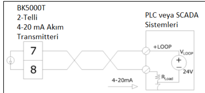
Şekil 7: BK 5000-T 4-20 mA Akım Transmitteri Kablolama Şeması
