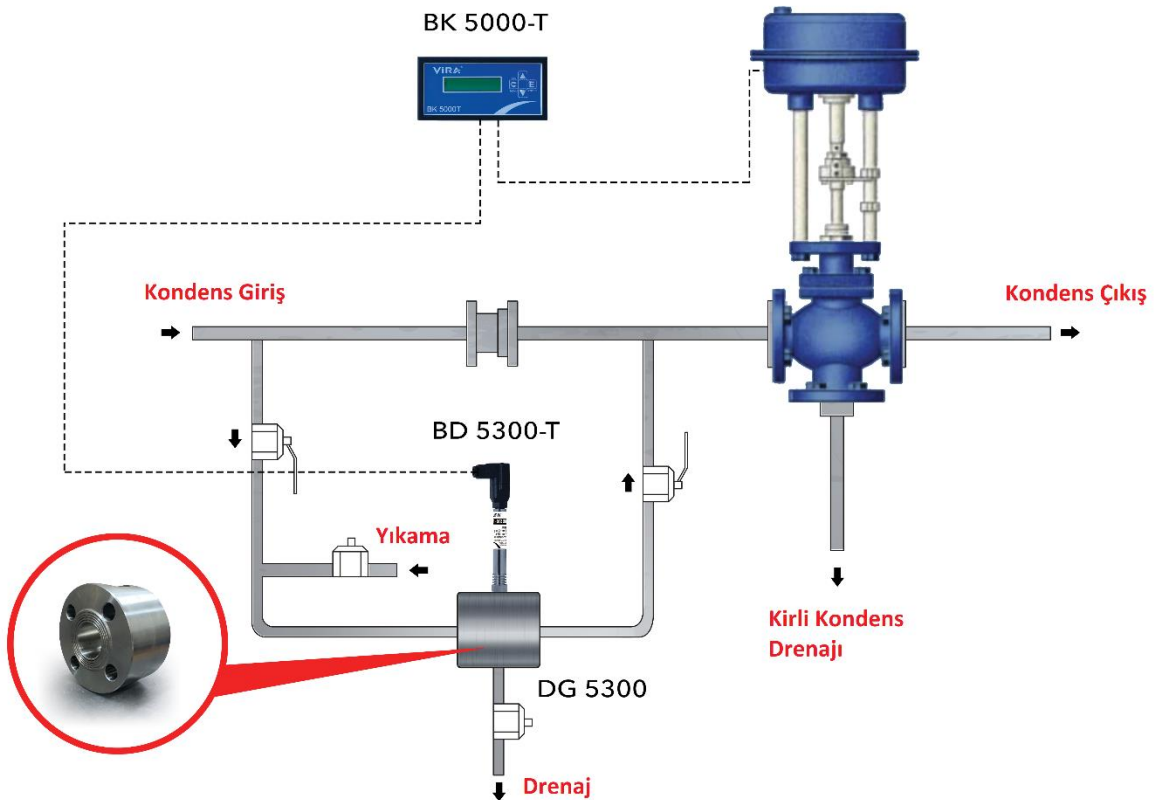
Şekil 1: Yüzey Blöf Sistemi BS3-T'nin buhar kazanına bağlantı şekli
