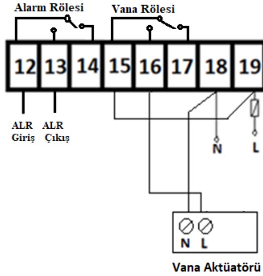
Şekil 6: BK 5000-T ve Vana Kablolama Şeması
